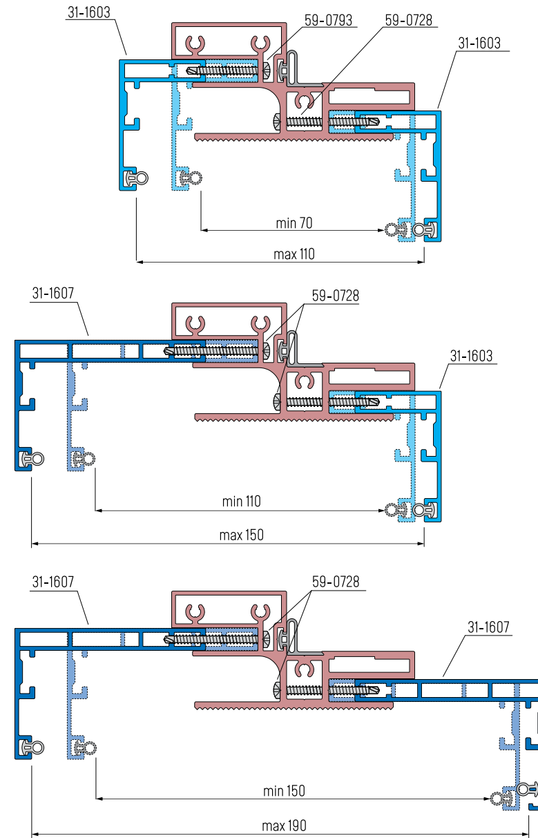
ADJUSTABLE DOOR FRAME - RANGES
