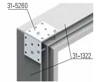
door frame
